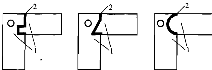
图2 法兰密封垫接头
