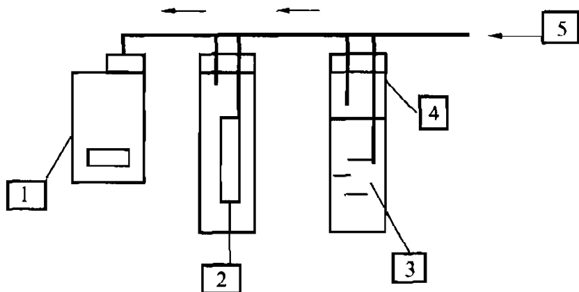
图 H. 3. 2 撞击采样法示意
