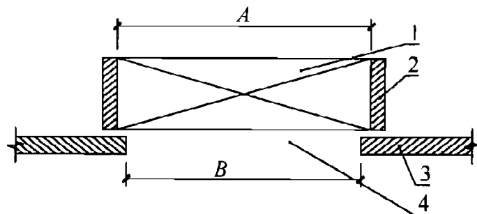
图 5.6.6 过滤器安装尺寸
