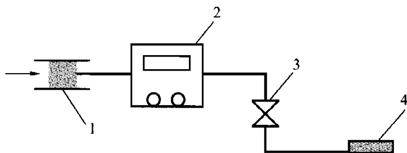
图 H. 4. 1 吸附管采样法示意
