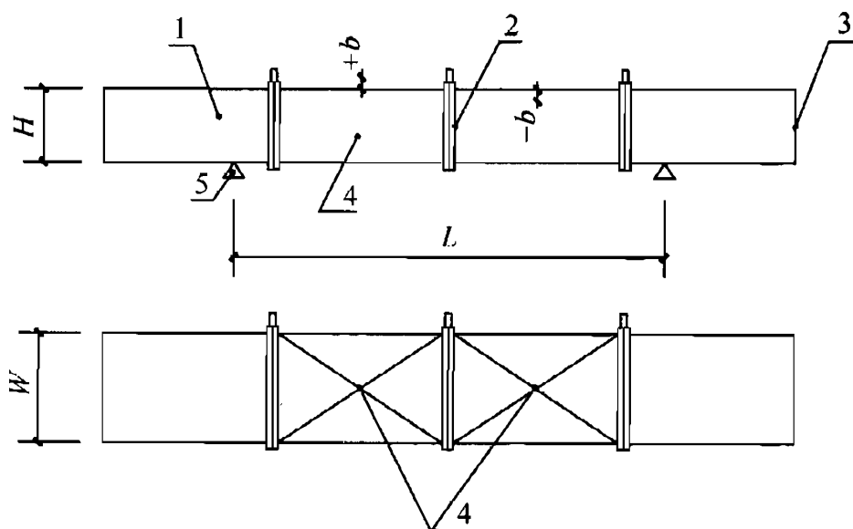
图 5.7.2-1 风管管壁变形
