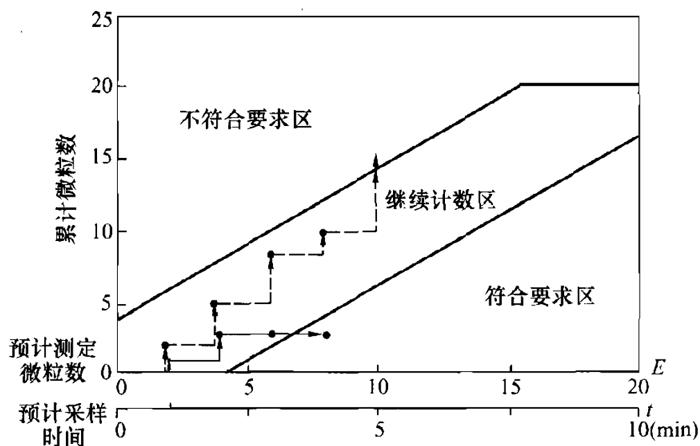
图 E. 4. 2 顺序采样法判断范围
