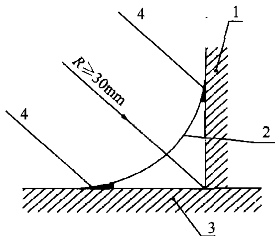
图 4.5.2 型材过渡墙角的圆弧做法
