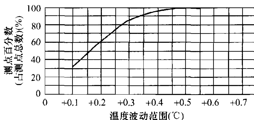
图 E. 5. 2-1 温（湿）度波动曲线
