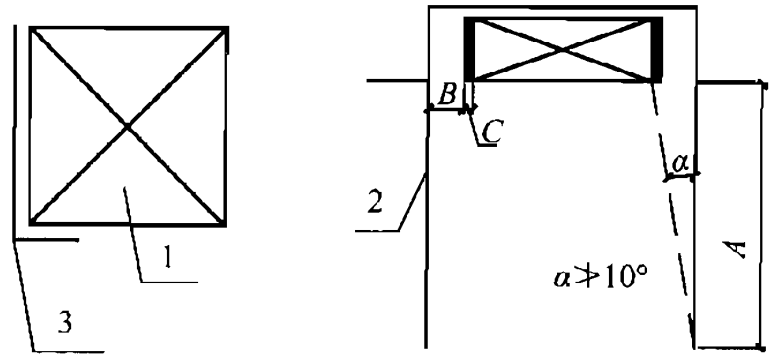
图 D. 3. 10 检漏用挡板或围挡管
