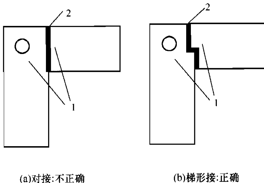
图 5.3.3 法兰密封垫接头
