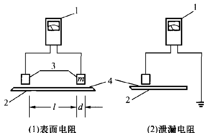
图 E. 9. 3 表面导静电性能测试装置
