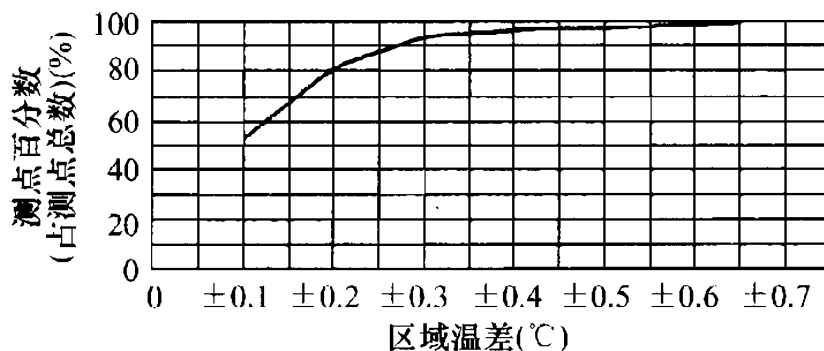
图 E.5.2-2 区域温（湿）差曲线
