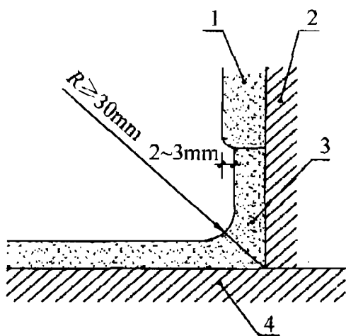
图 4.5.1 整体墙角的圆弧做法
