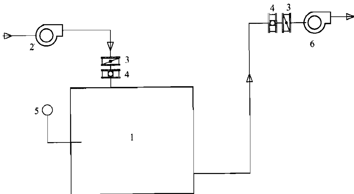
图 G. 2.1 压力衰减法系统
