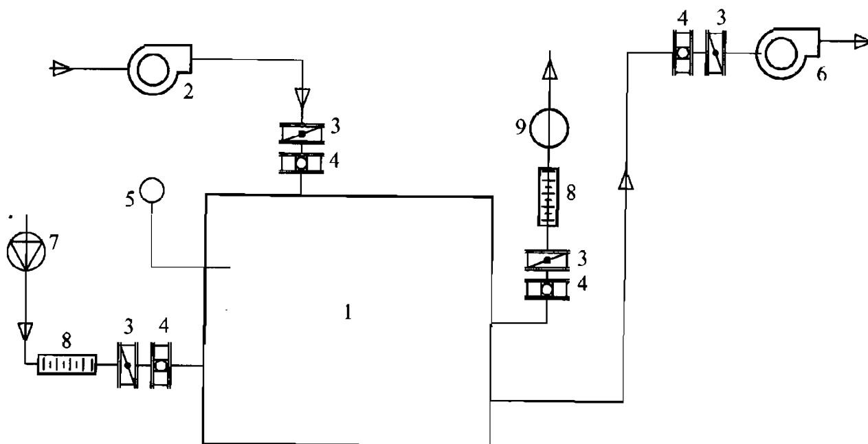
图 G.3.1 恒压法测试系统
