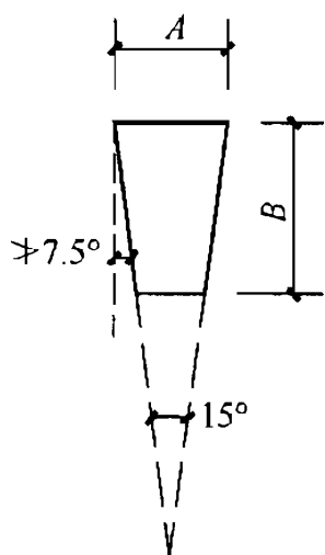
图 E. 1. 7 锥形套风管
