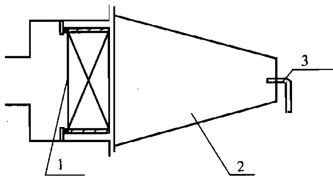
图 F.1.1 套筒结构示意图
