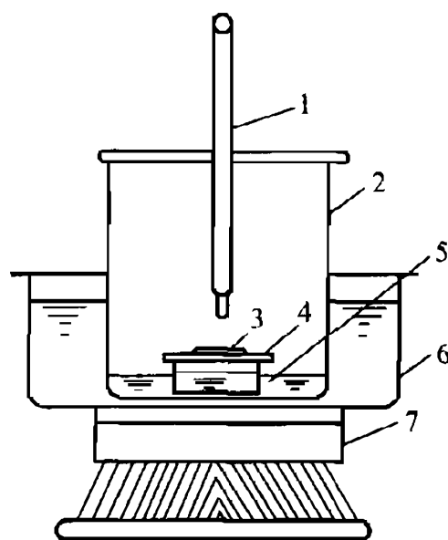
图 E.4.4 滤膜制片装置示意
