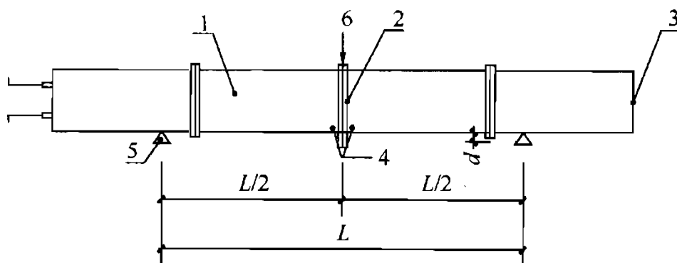
图 5.7.2-2 风管挠度变形
