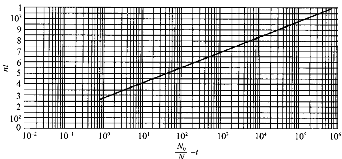
图 E. 11.3 乱流洁净室自净时间计算图
